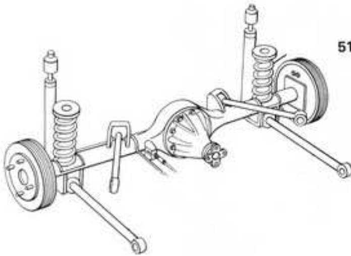
MODEL 510 S.W. ( '69-73)
