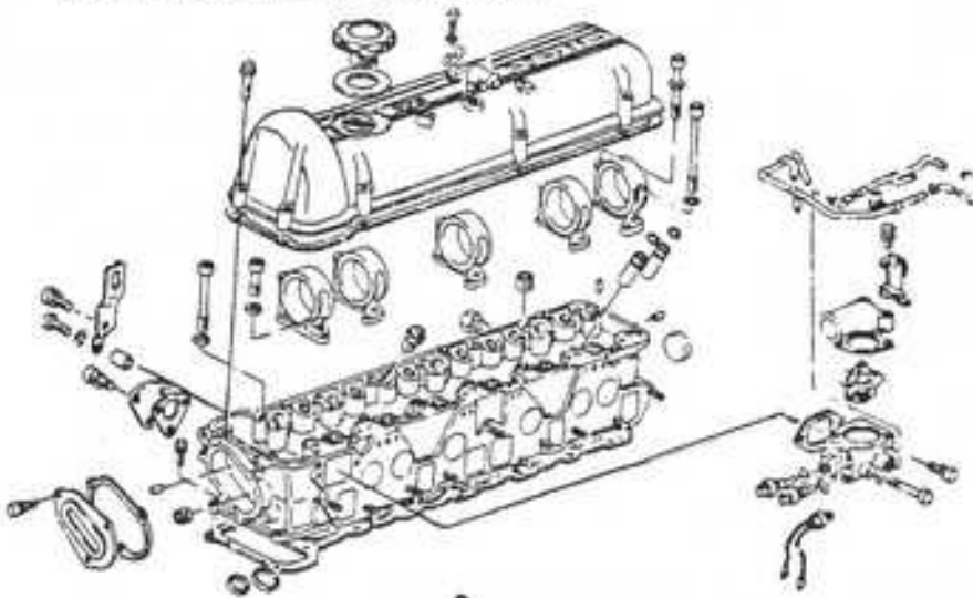
L-28E (280Z), L-24E (810) Typical
